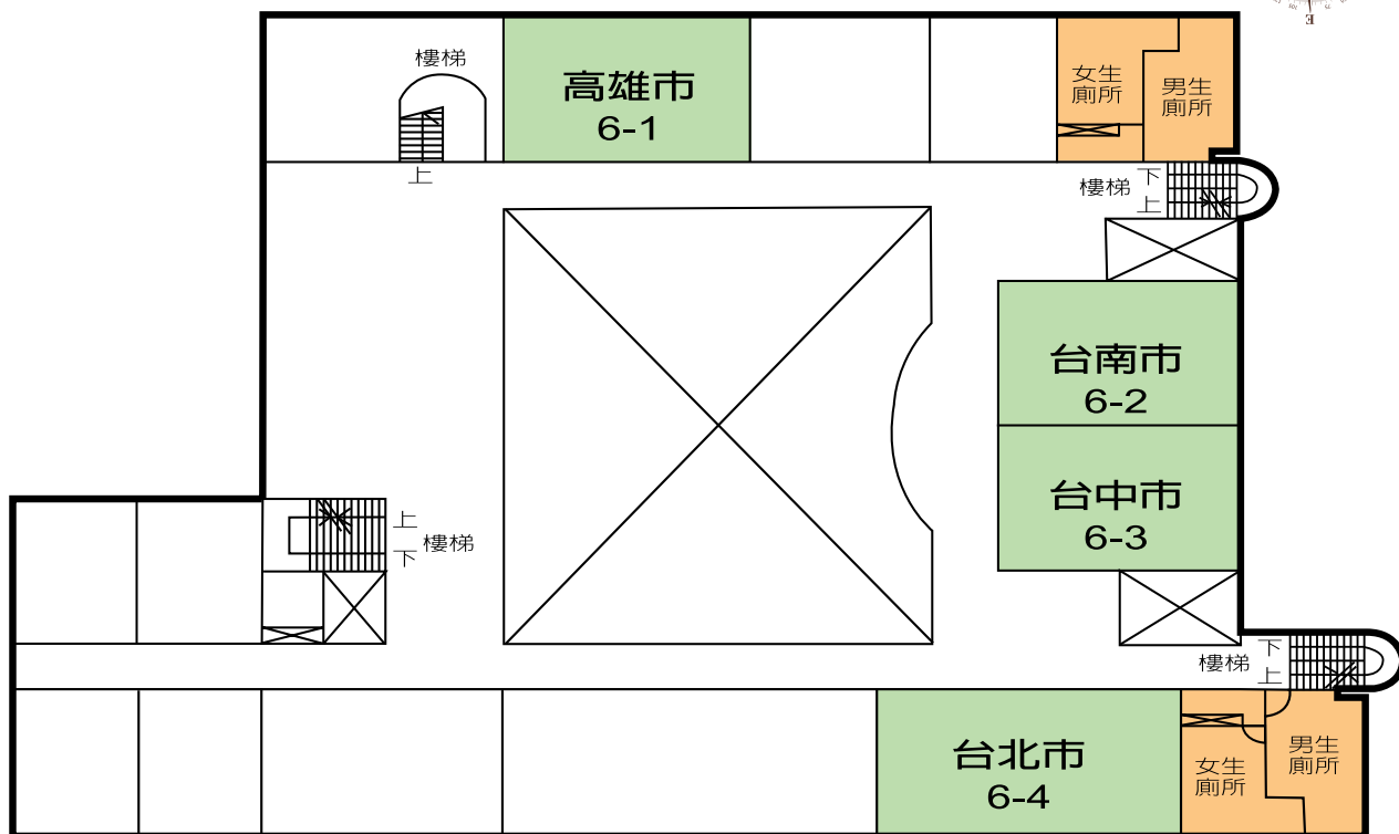
(宜蘭大學)經德大樓地下一樓平面圖
