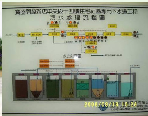
污水處理系統
