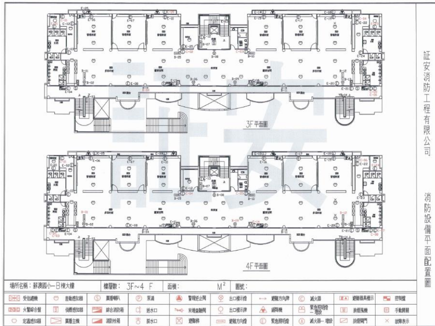
圖 6-2-4、B 棟 3F~4F 消防安全設施配置圖
