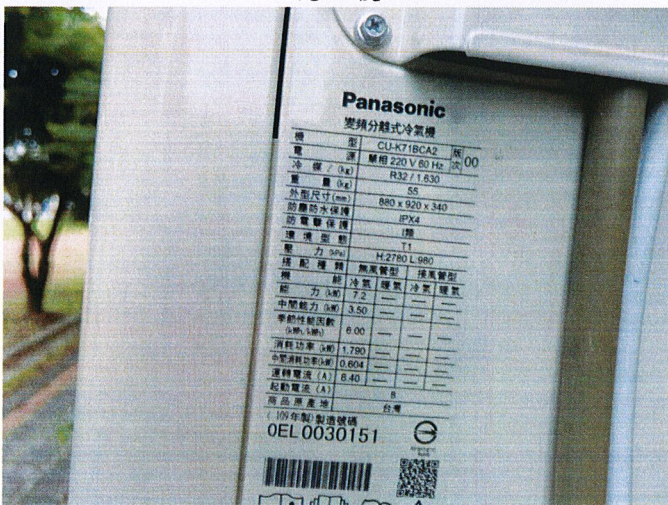
※無風管空調機提供新室外機(製造號碼)照片
